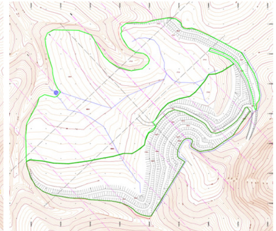
Vista en planta de una explotación de calizas, en la cuales se podrá actuar sobre la plaza de cantera generada y los taludes restaurados en la zona NE.
