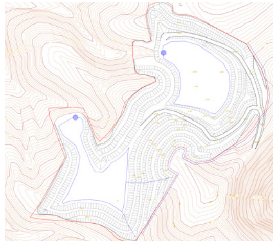
Vista en planta de una explotación de calizas, en la cual se podría actuar sobre la plaza de cantera generada y los taludes restaurados en la zona NE (al poseer una adecuada orientación)
