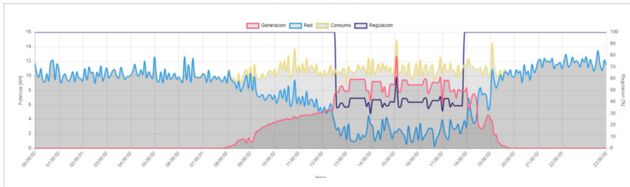
ILUSTRACIÓN 22: Gráfica vertido 0
